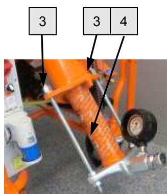
Рис. 87: Замена насоса
