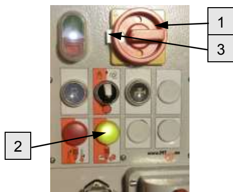
Рис. 38: Включение
