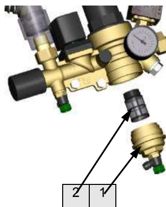
Рис. 100: Грязеулавливающая сетка
