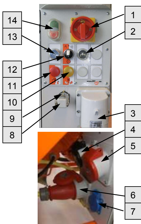
Рис. 7: Распределительный шкаф
