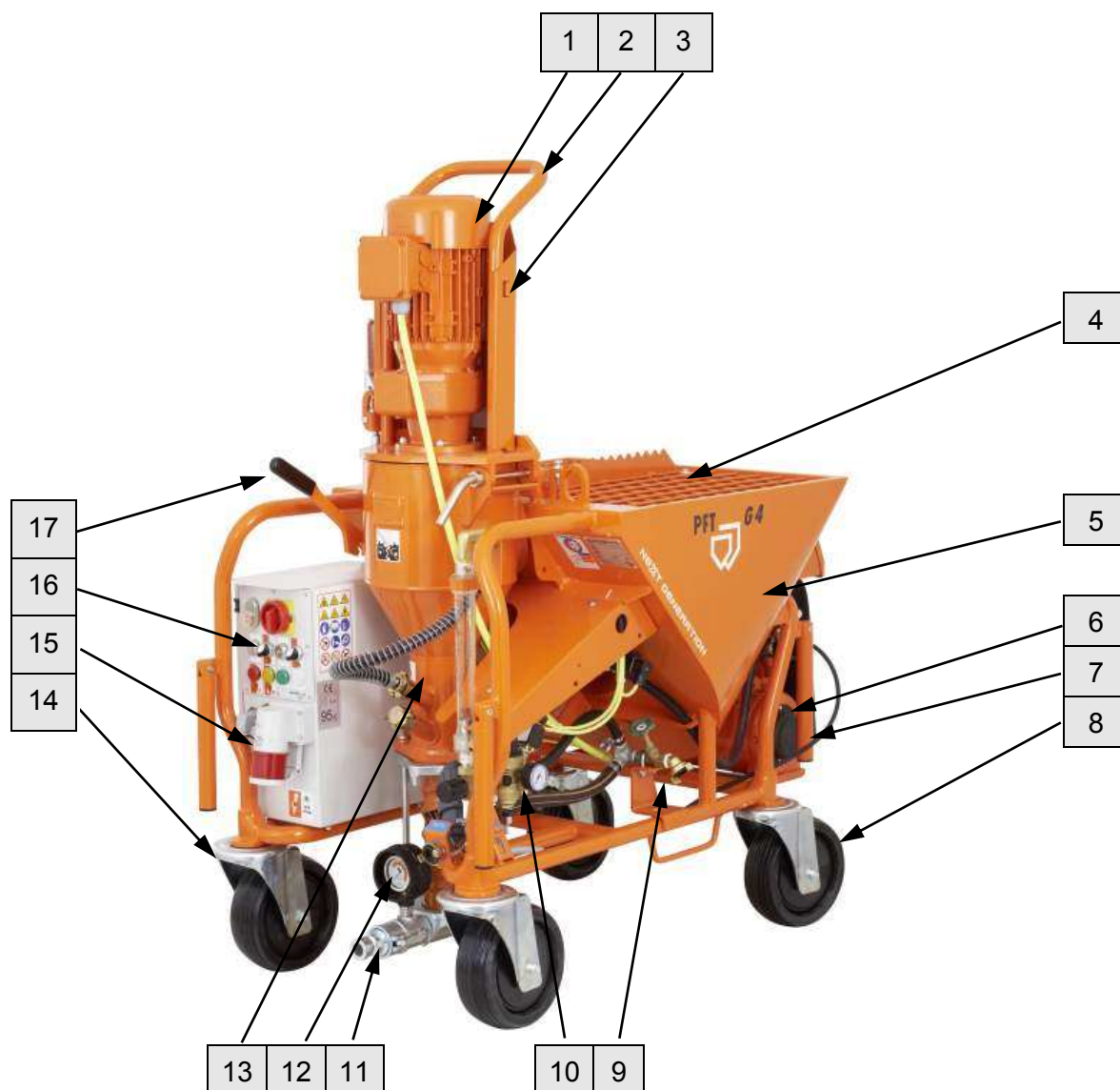
Рис. 5: Обзор узлов
