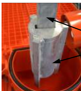
Рис. 81: Установка очистителя смесительной башни
