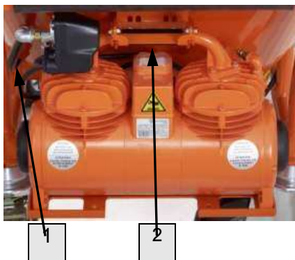
Рис. 96: Воздушный компрессор
