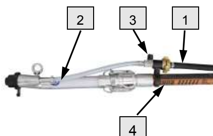
Рис. 56: Растворный пистолет
