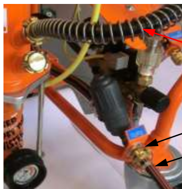
Рис. 35: Подключение воды
