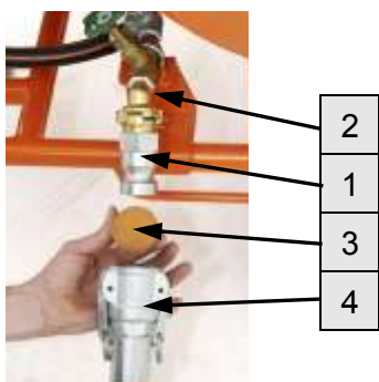
Рис. 77: Очистка рукава подачи раствора
