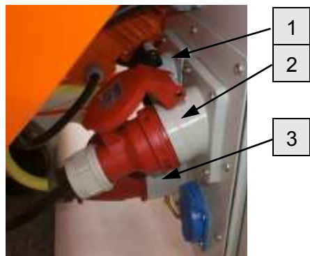
Рис. 33: Электрические подключения
