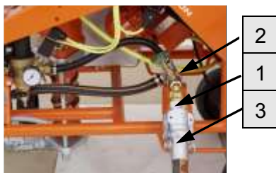
Рис. 52: Подготовка рукава для подачи раствора
