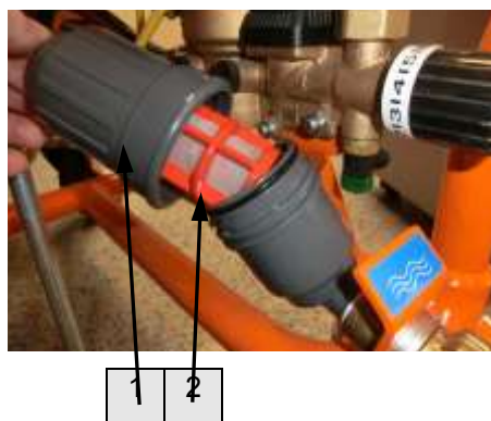
Рис. 99: Очистка сетки
