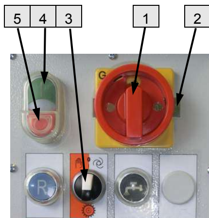
Рис. 73: Изменение направления вращения
