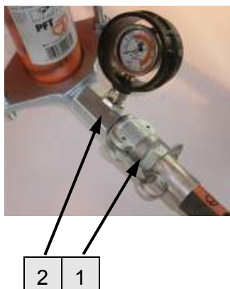
Рис. 53: Подключение рукава для подачи раствора
