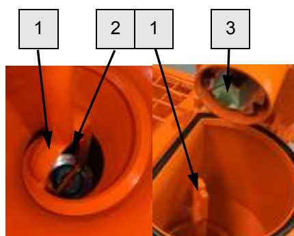
Рис. 85: Установка смесительной спирали
