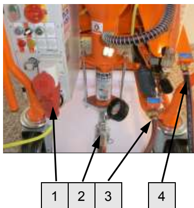
Рис. 11: Вводы
