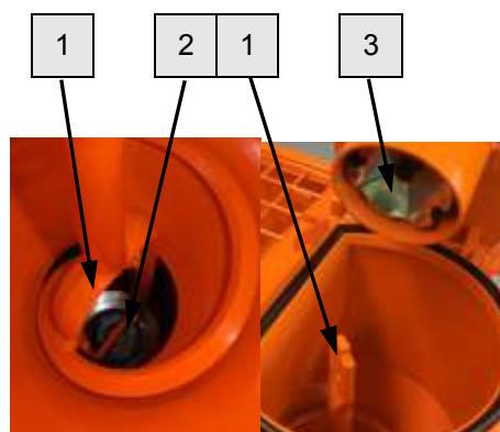
Рис. 98: Установка смесительной спирали
