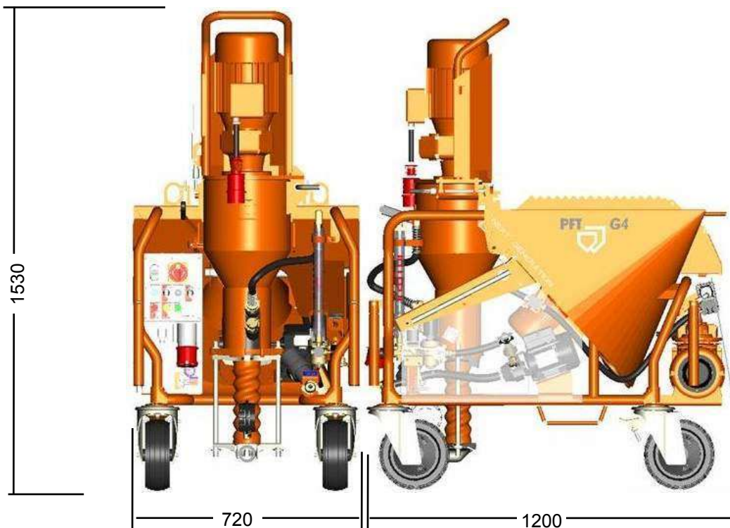
Рис. 2: Габаритный чертеж
