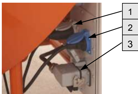
Рис. 38: Электрические подключения
