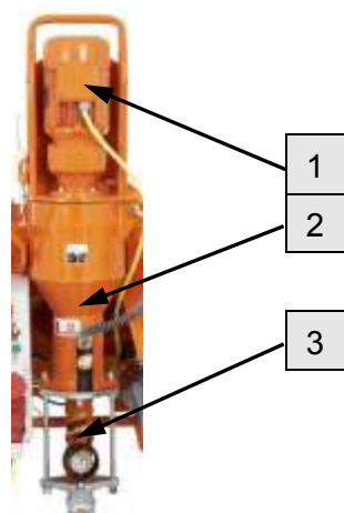
Рис. 8: Смесительная башня с приводом и насосом
