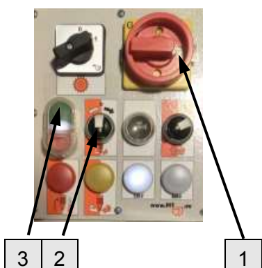
Рис. 78: Изменение направления вращения (230 В)
