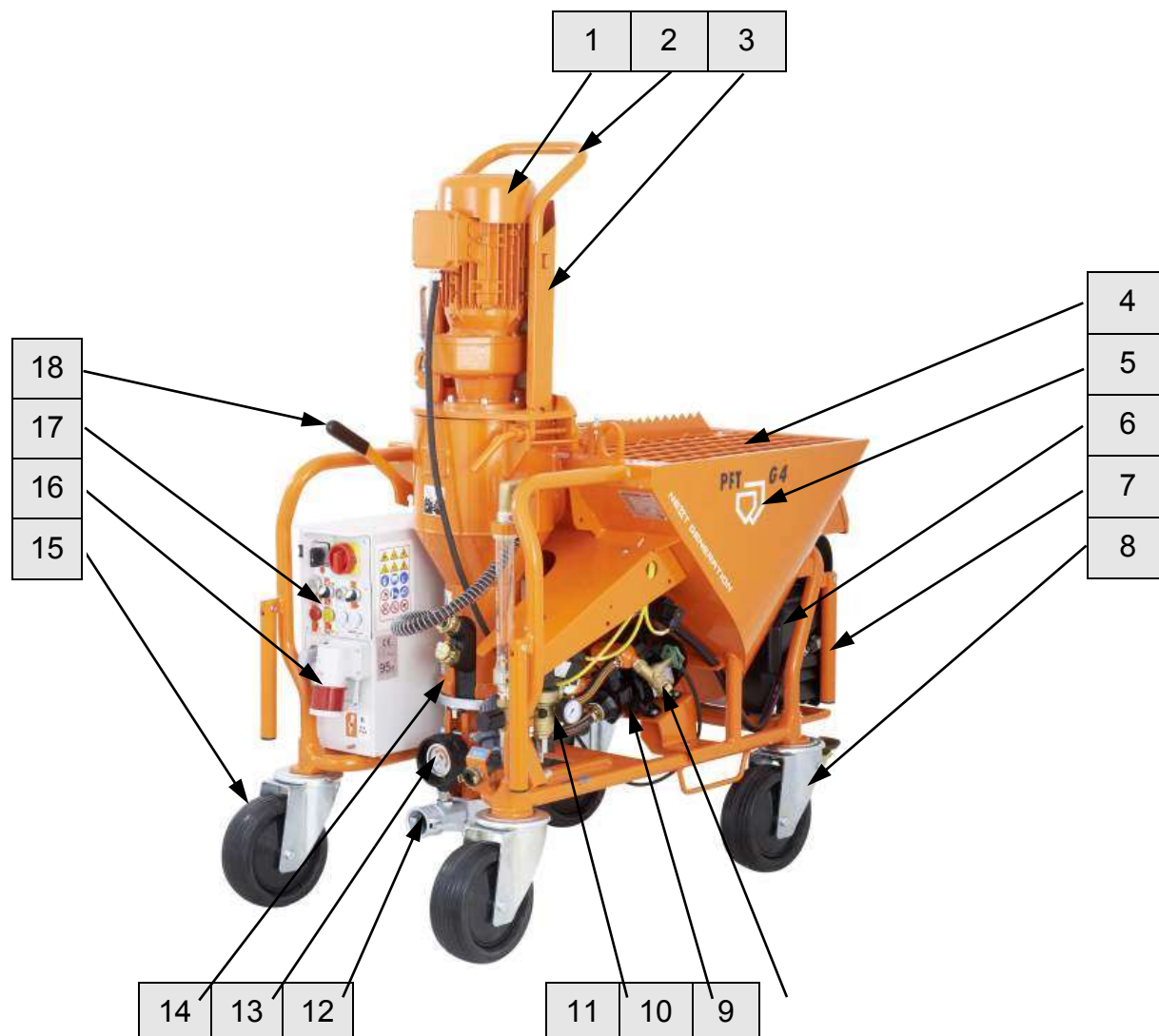
Рис. 5: Обзор узлов
