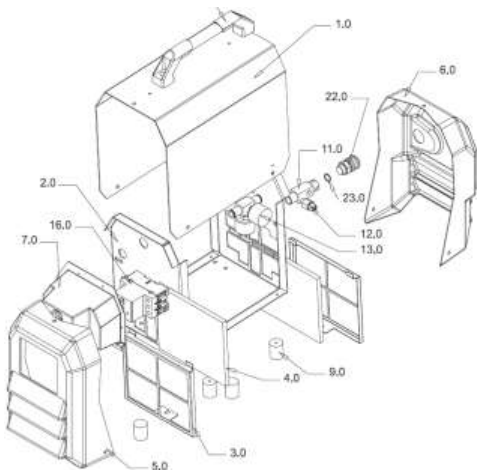
Рис. 109: Фильтровальная рама
