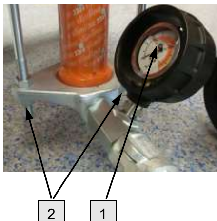
Рис. 73: Проверка давления раствора
