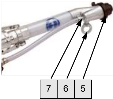
Рис. 91: Трубка воздушного сопла и насадка растворного пистолета
