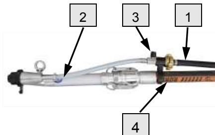
Рис. 62: Растворный пистолет
