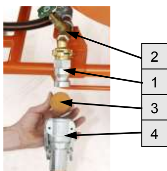
Рис. 90: Очистка рукава подачи раствора
