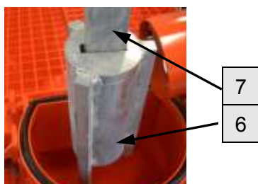
Рис. 97: Снятие очистителя смесительной башни
